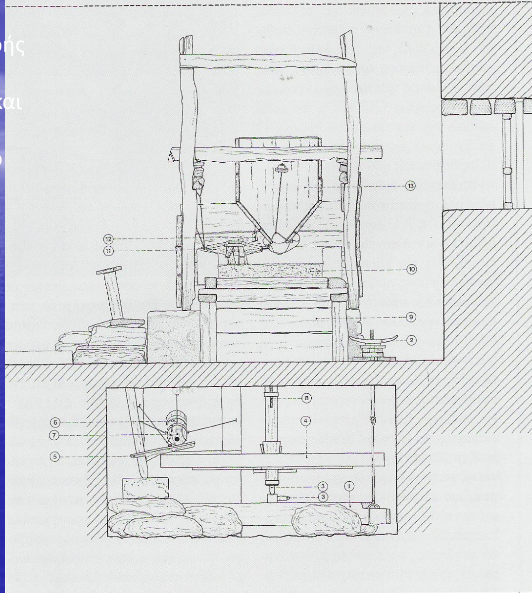
Εικ. 70. Ο νερόμυλος της Σαμοθράκης (ο μηχανισμός του νερόμυλου της Μ. Μπαλκανίου στα Αλώνια). 1. ταμπανόξυλο, 2. σταυρός, 3. βελόνια, 4. φτερωτή, 5. σπριματήρα, 6. ζουρνάς, 7. αξιά, 8. άξονας, 9. ταμπάνι-αλευροδόχη, 10. ταμπάνι-ελαστήρας, 11. βελόνια, 12. κουδουνάκι, 13. κοφινίδα.
