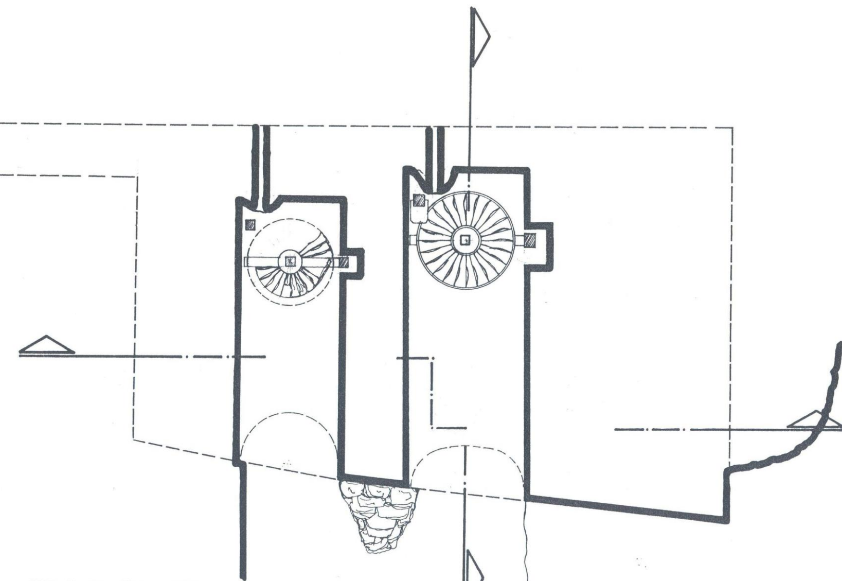
ΚΑΤΟΨΗ ΣΤΑΘΜΗΣ ΦΤΕΡΩΤΩΝ
